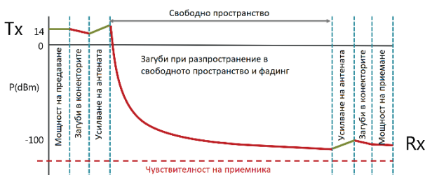
Фиг. 2. Определяне на енергийния бюджет на връзката
